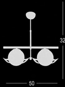
353-2 2xE27 Max.40W
