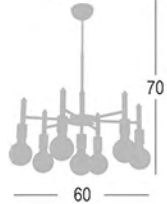
2077-7 7xE27 Max.60W
