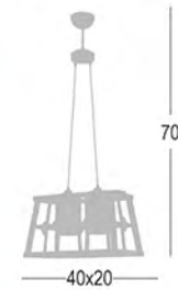
6099-2 2xE27 Max.60W
