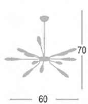
3011-12 12xE14 Max.40W
